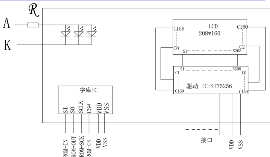
图 2: JLX208160G-9812-PL 电路框图
