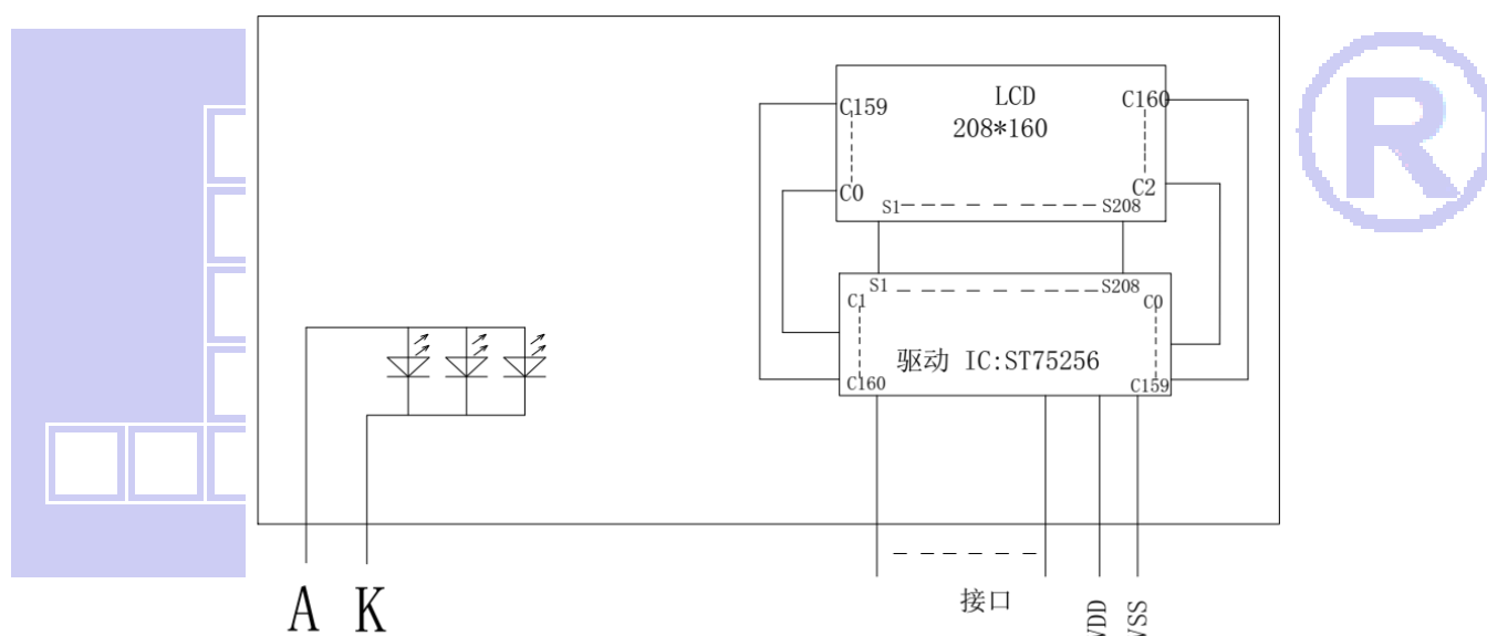
图 2: JLX208160G-9812-PN 图像点阵型液晶模块的电路框图
