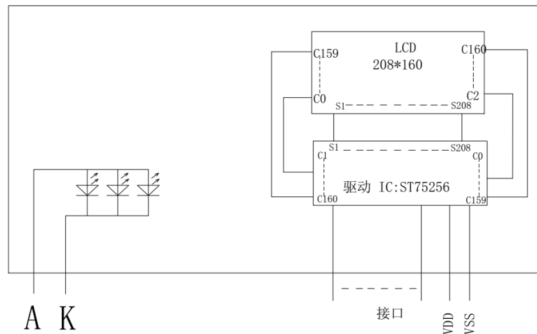
图 2: JLX208160G-9812-BN 图像点阵型液晶模块的电路框图
