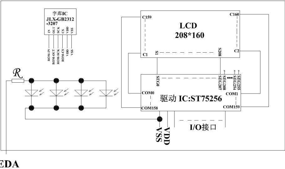
图 2: JLX208160G-9813-PL 电路框图
