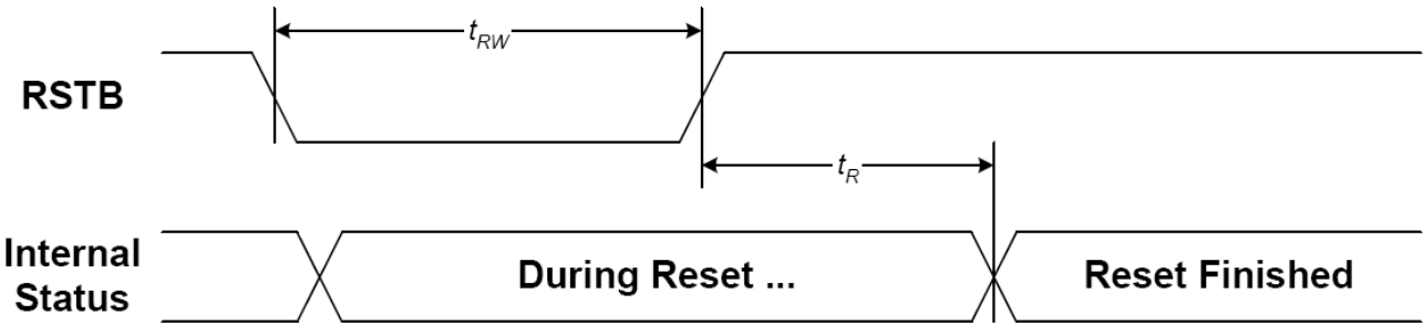
图 7：电源启动后复位的时序
