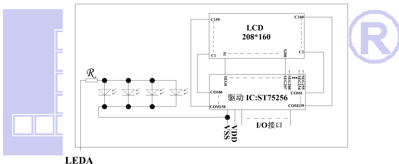
图 2：JLX208160G-9813-PN 图像点阵型液晶模块的电路框图
