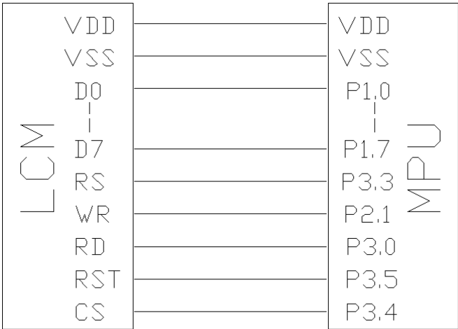
图 8: 并行接口图
