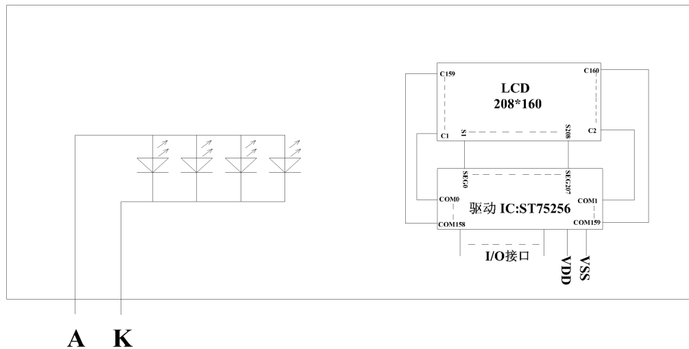
图 2: JLX208160G-9813-BN 图像点阵型液晶模块的电路框图
