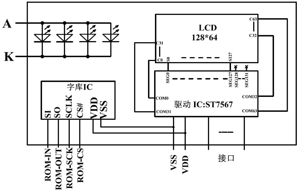
图 2: 电路框图
