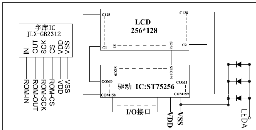
图 2: JLX256128G-978-PL 电路框图
