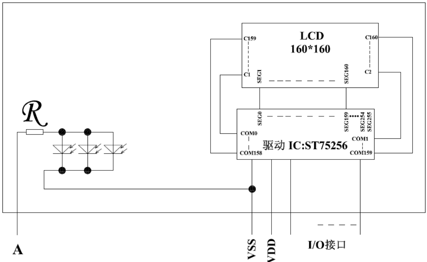
图 2: JLX160160G-979-PN 图像点阵型液晶模块的电路框图
