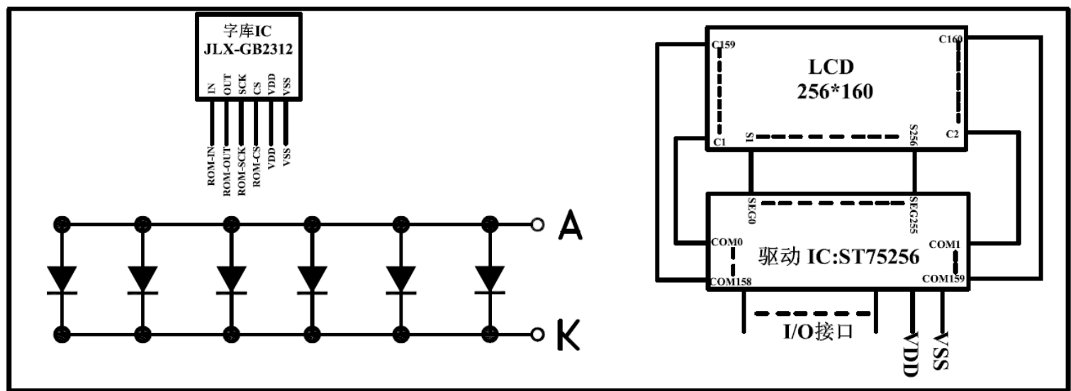
图 2: JLX256160G-680-PL 电路框图
