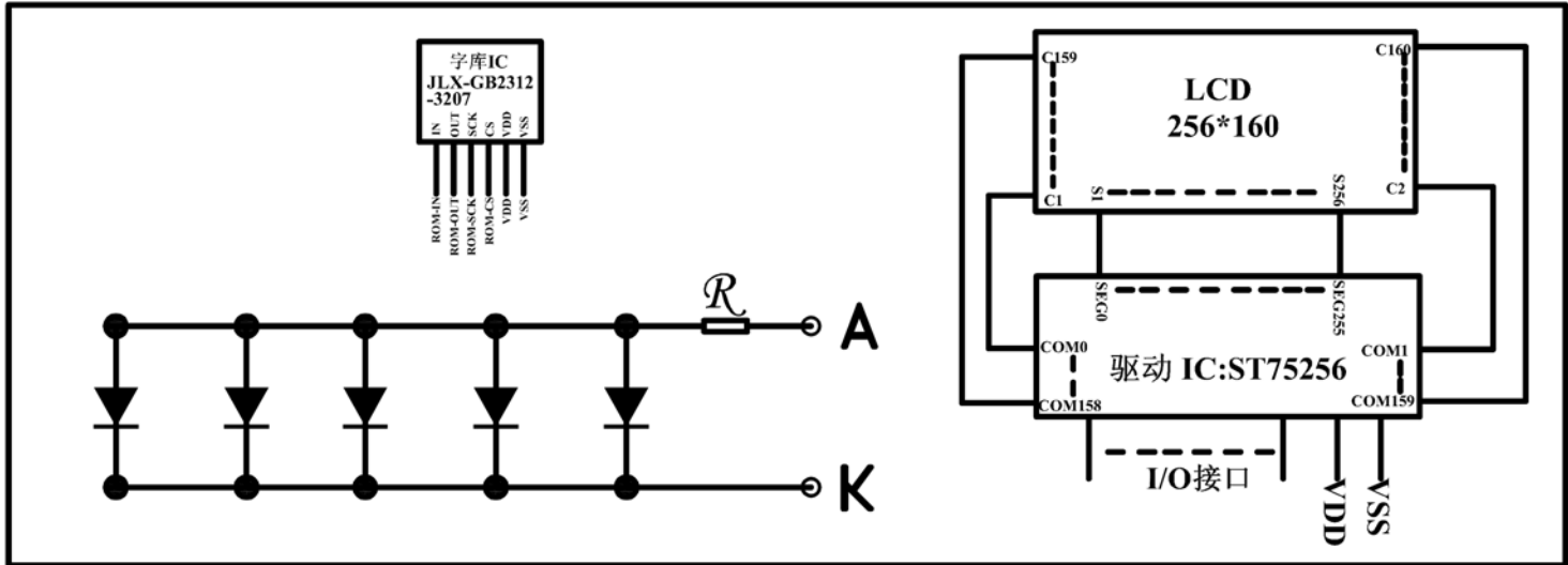
图 2: JLX256160G-91002-PL 电路框图
