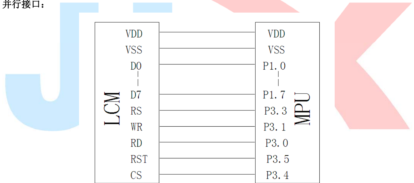
图 9. 并行接口
