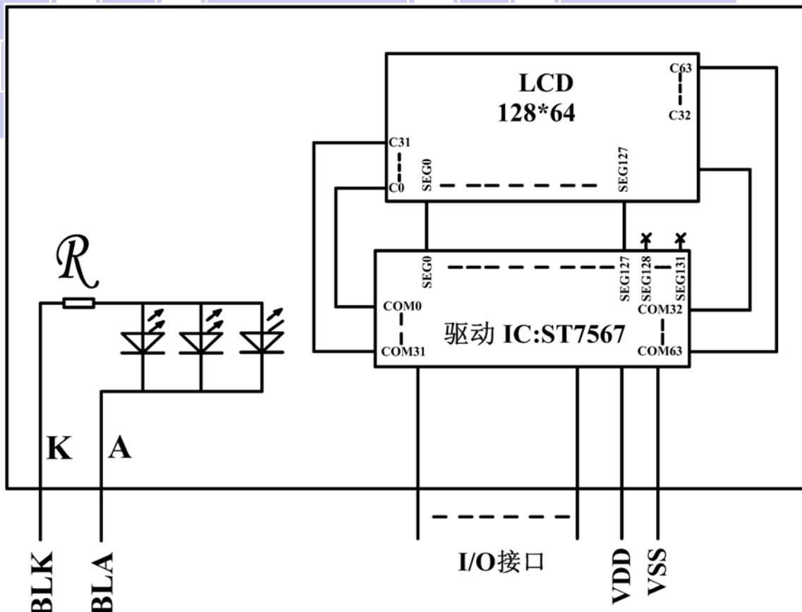
图 2: JLX12864G-330-PN 图像点阵型液晶模块的电路框图
