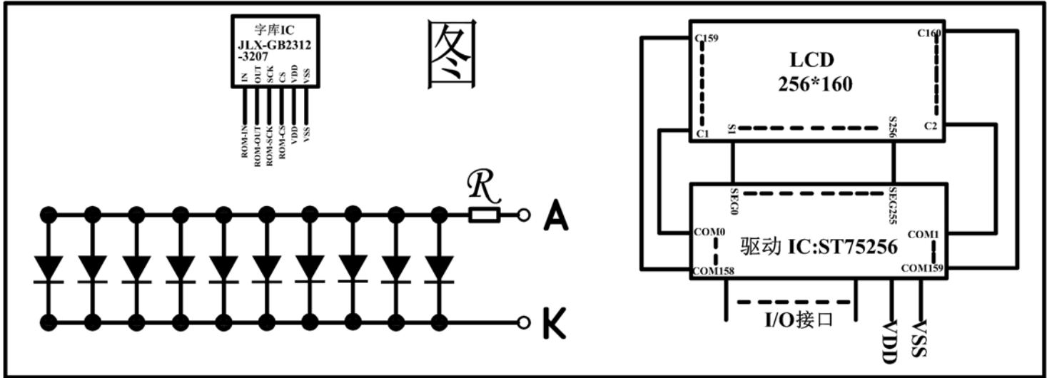
图 2: JLX256160G-922-PL 电路框图
