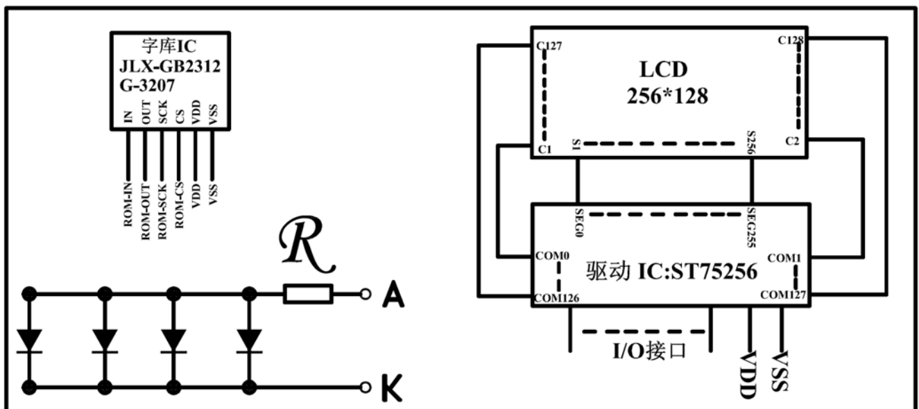
图 2: JLX256128G-92002-PL 电路框图
