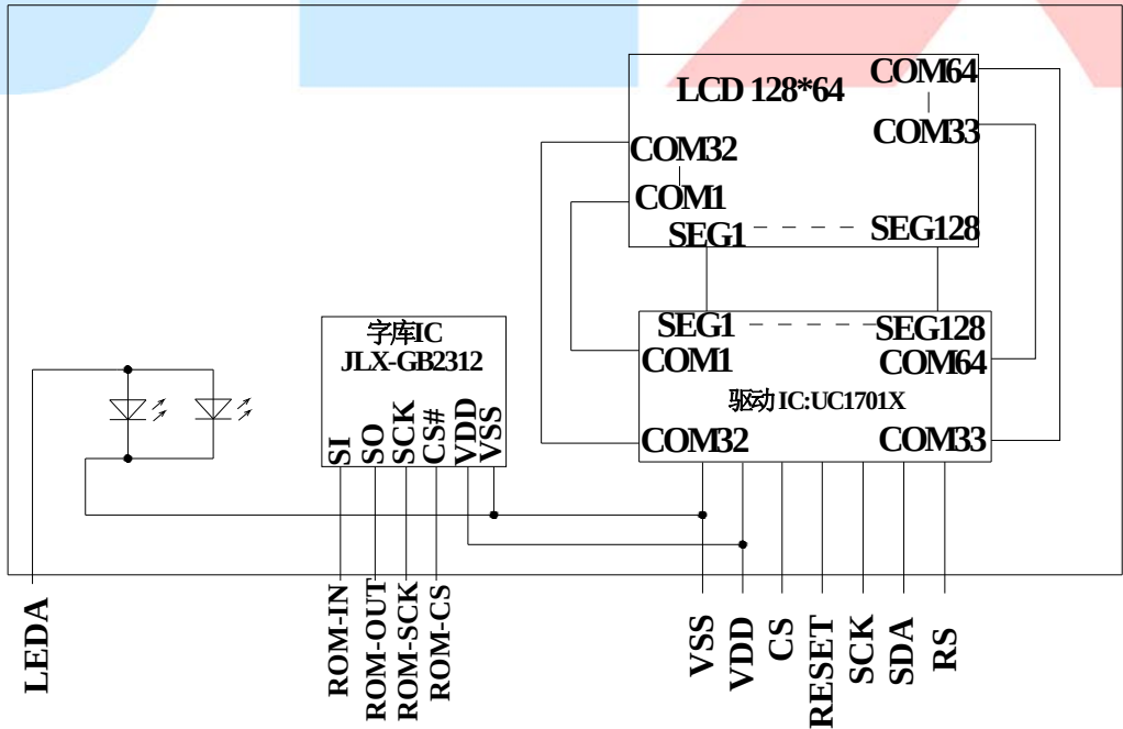
图 2：电路框图
