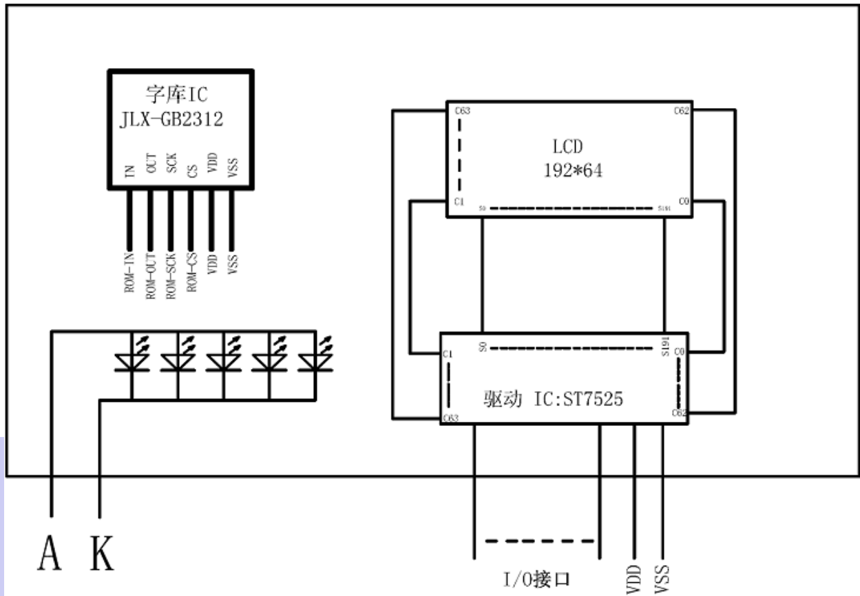
图 2: 电路框图
