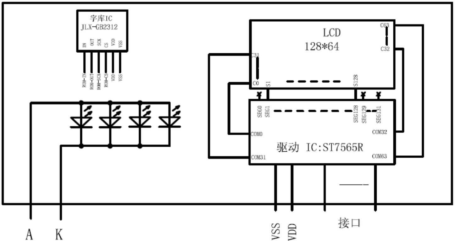
图 2: 电路框图
