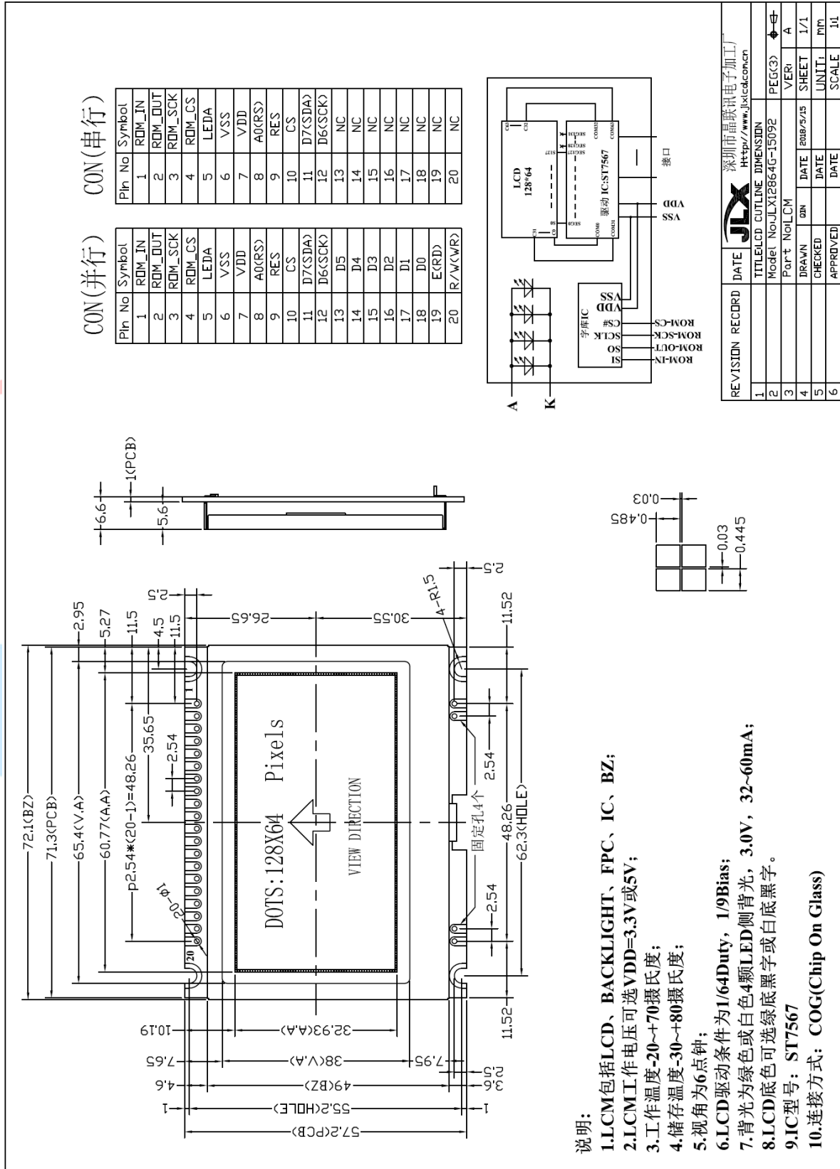
图 1. 外形尺寸
