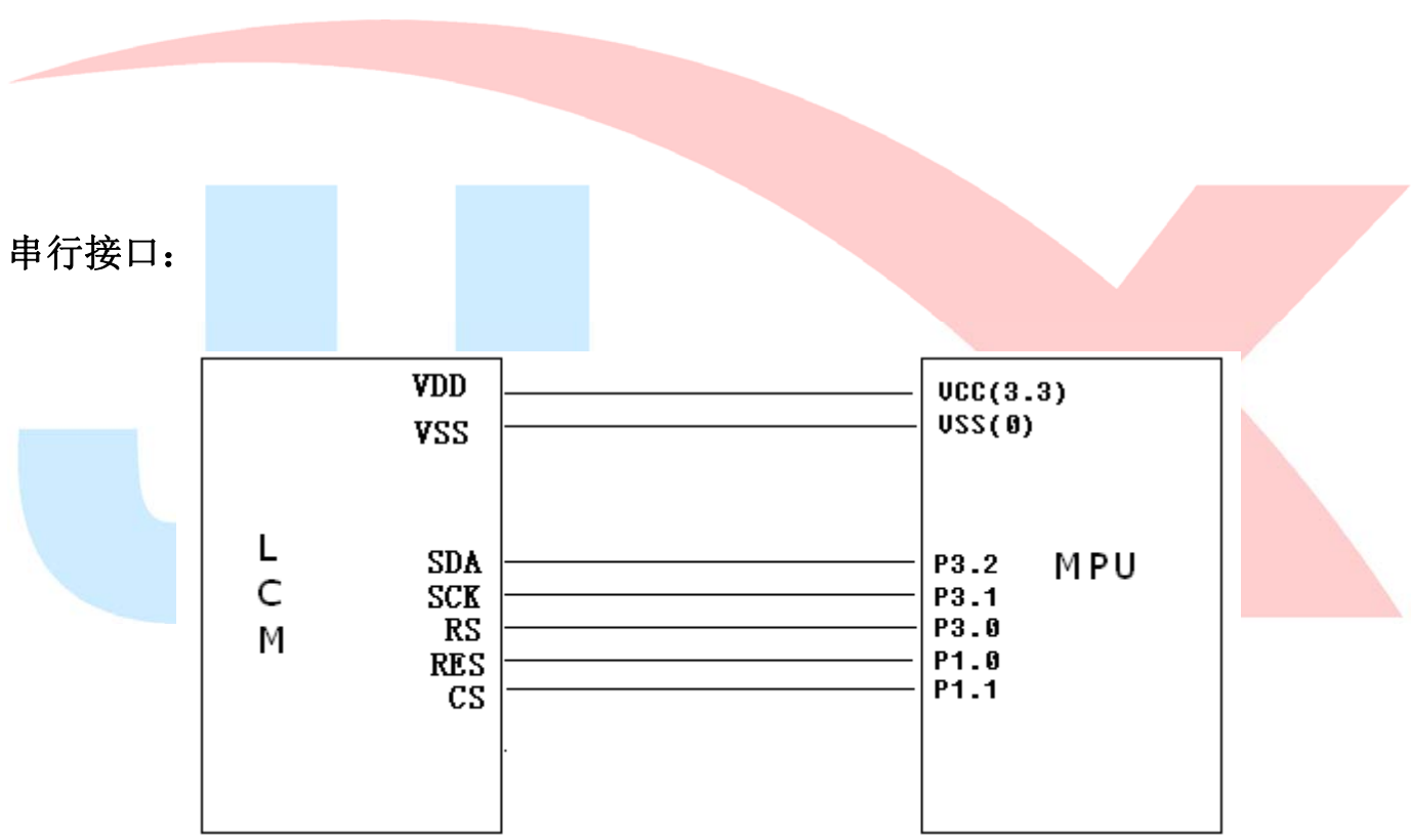
图 9. 串行接口
