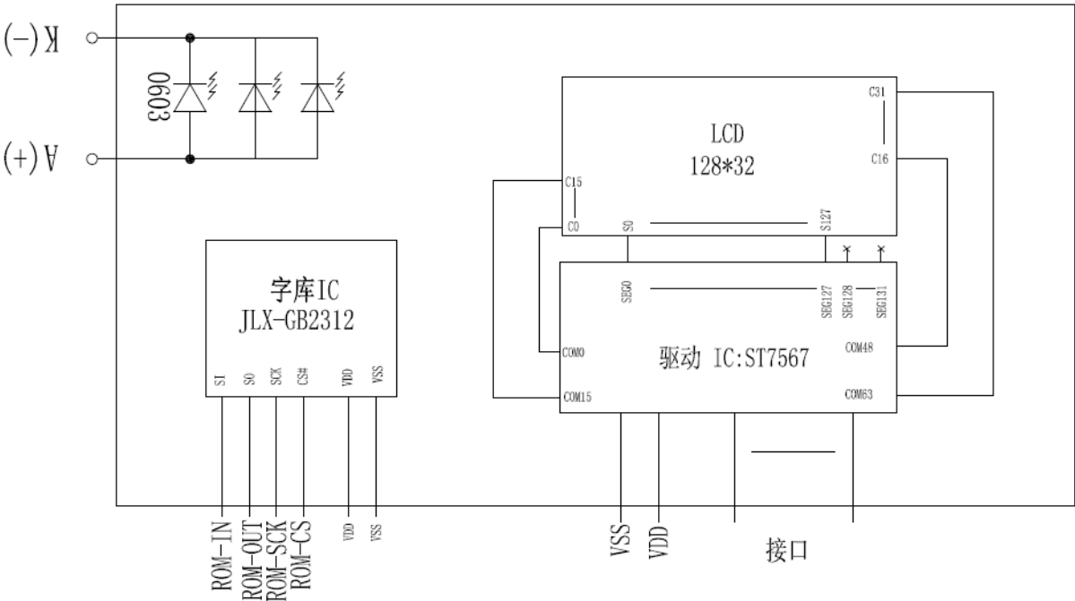
图 2: 电路框图
