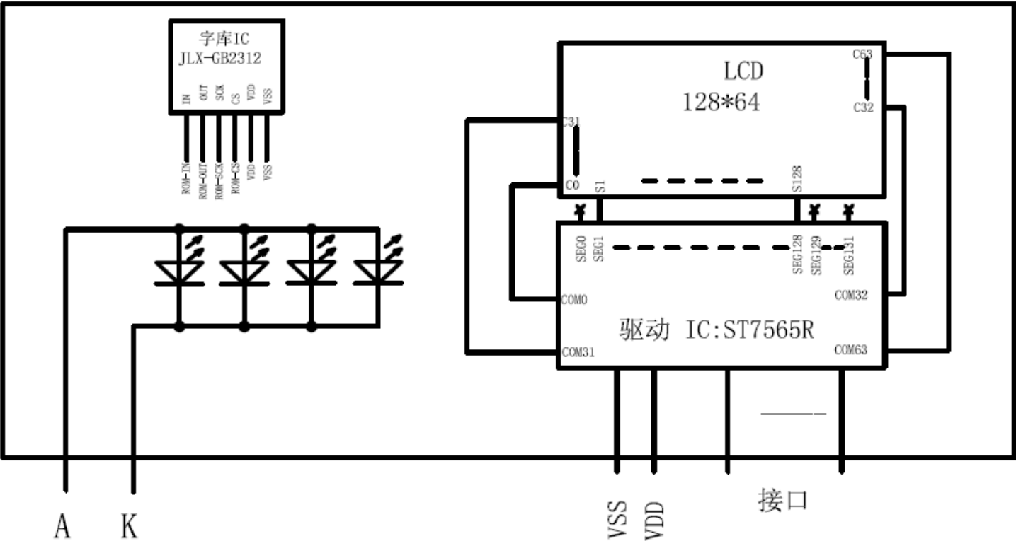
图 2: 电路框图
