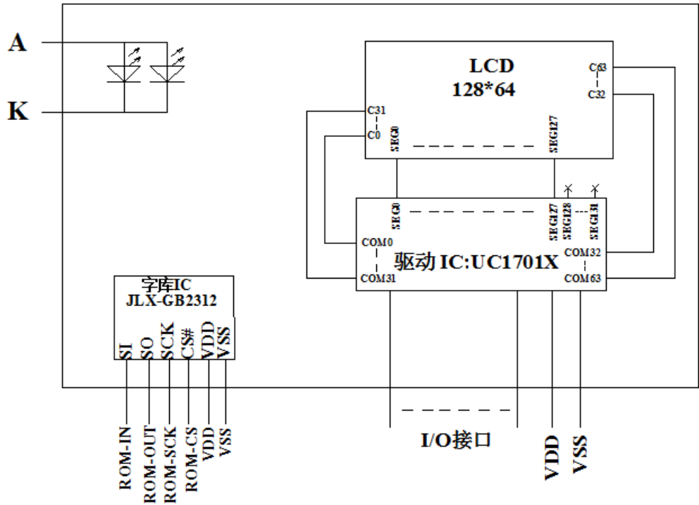
图 2: 电路框图
