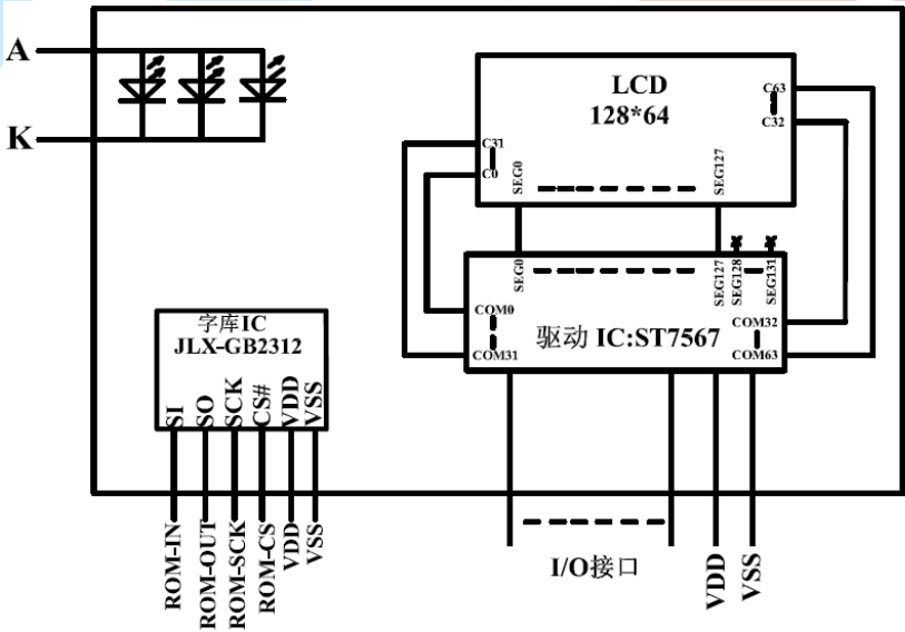
图 2: JLX12864G-33206 电路框图
