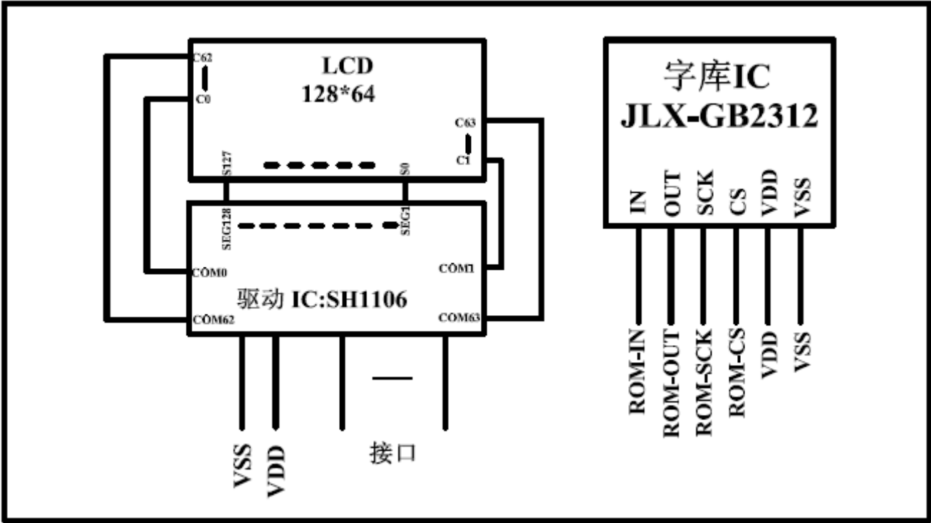
电路框图
